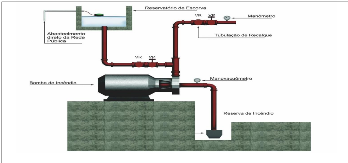
Figura C.3: Exemplo de afogamento de bomba de incêndio
