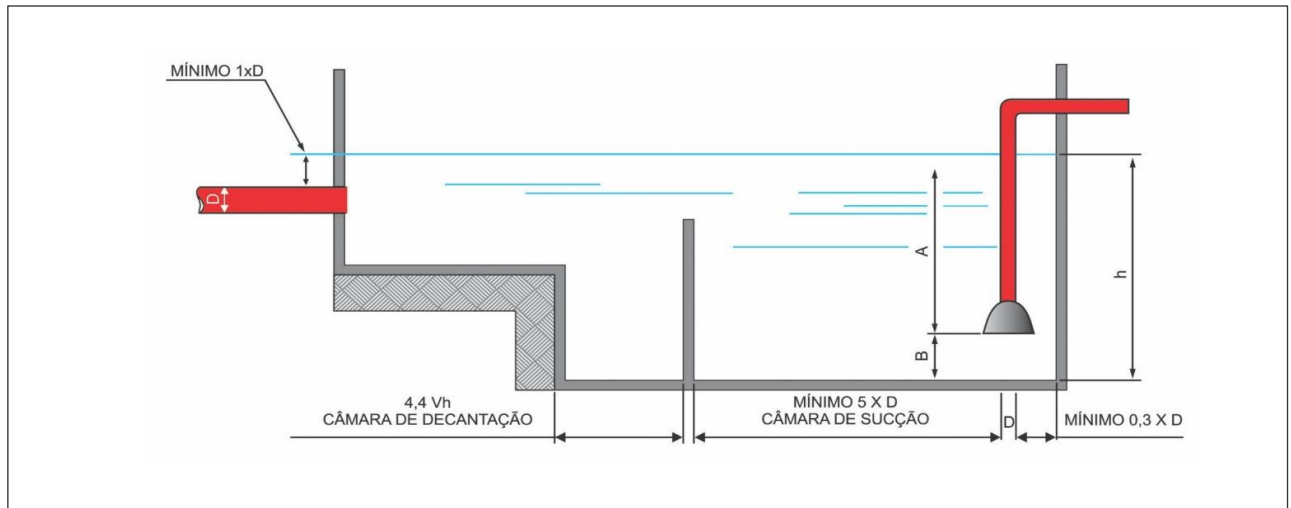
Figura B.6 - Alimentação natural de reservatório por conduto
