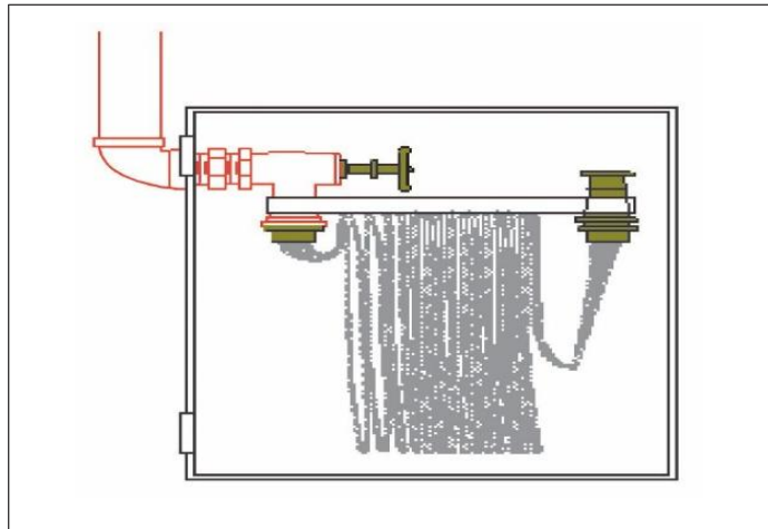
Figura 3: Suporte para mangueira tipo “rack”
