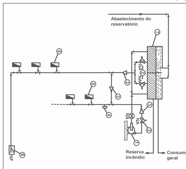
Figura C.6: Esquema de instalação de bomba de reforço abastecendo os pontos de hidrantes ou mangotinhos mais desfavoráveis considerados no cálculo, (prumada específica)
