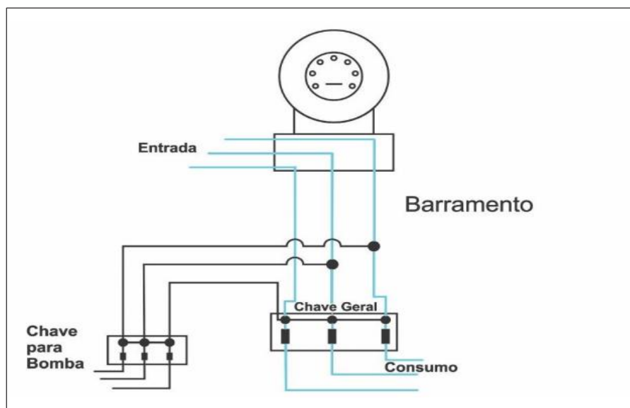
Figura C.4: Esquema de ligação elétrica para acionamento da bomba de incêndio
