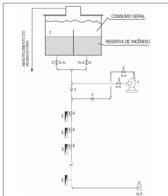
Figura C.5: Esquema de instalação de bomba de reforço abastecendo os pontos de hidrantes ou mangotinhos mais desfavoráveis considerados no cálculo, por uma só prumada
