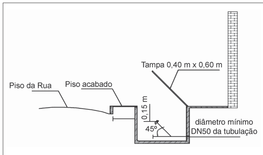
Figura 2: Dispositivo de recalque no passeio público
