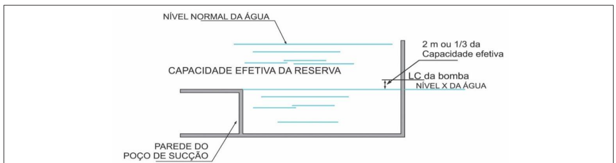
Figura C.1: Condição positiva de sucção da bomba de incêndio
