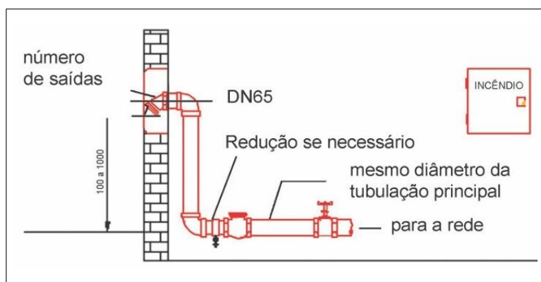
Figura 1: Dispositivo de recalque tipo coluna
